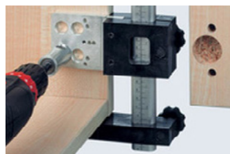
Центричен додаток за навртување на куки во сид
