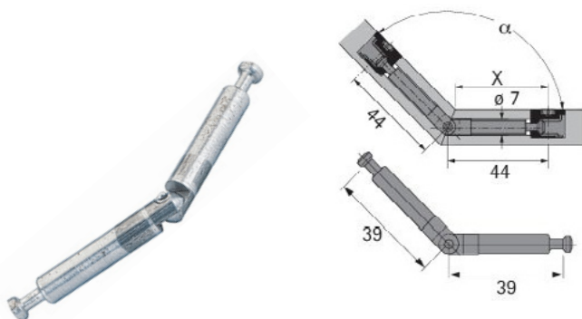
6643 | Аголен врзник за спојка 100°-160° | 39 x 39mm | 63 ден.
