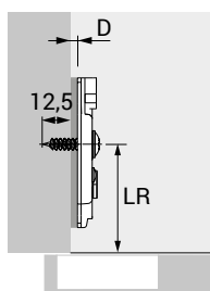
SYSTEM 8099 "Hettich Direkt" Подложка со штраф "Direkt" со штел
