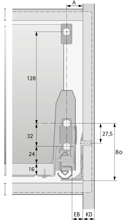
Бушење на фронт
