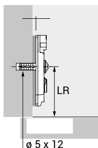
SYSTEM 8099 Подложка со типла и штраф со штел
