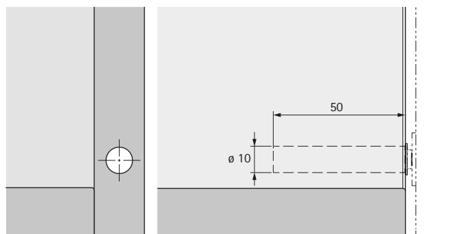
Шема за бушење за кратко водење
