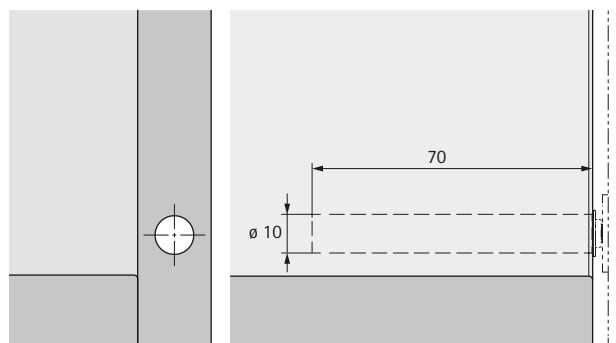
Шема за бушење за долго водење
