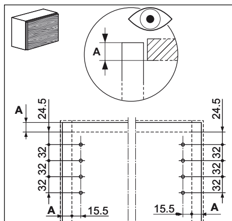
Предни конектори за дрвени панели и широки алуминиумски рамки
