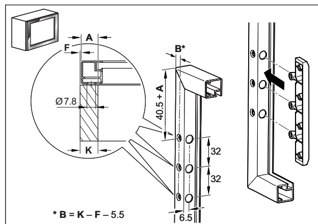
Предни конектори за 20mm алуминиумски рамки
