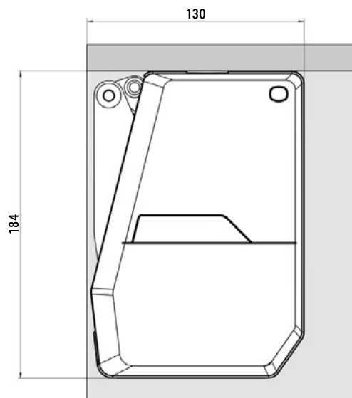
Левата страна со капакот
